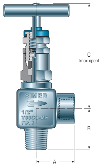
Mod. V08CS-MF
