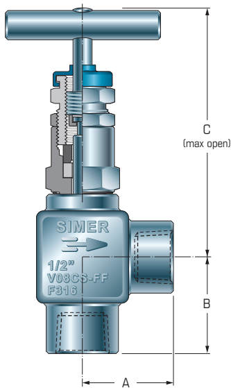
Mod. V08CS-FF
