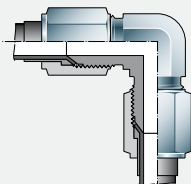
Gomito intermedio
